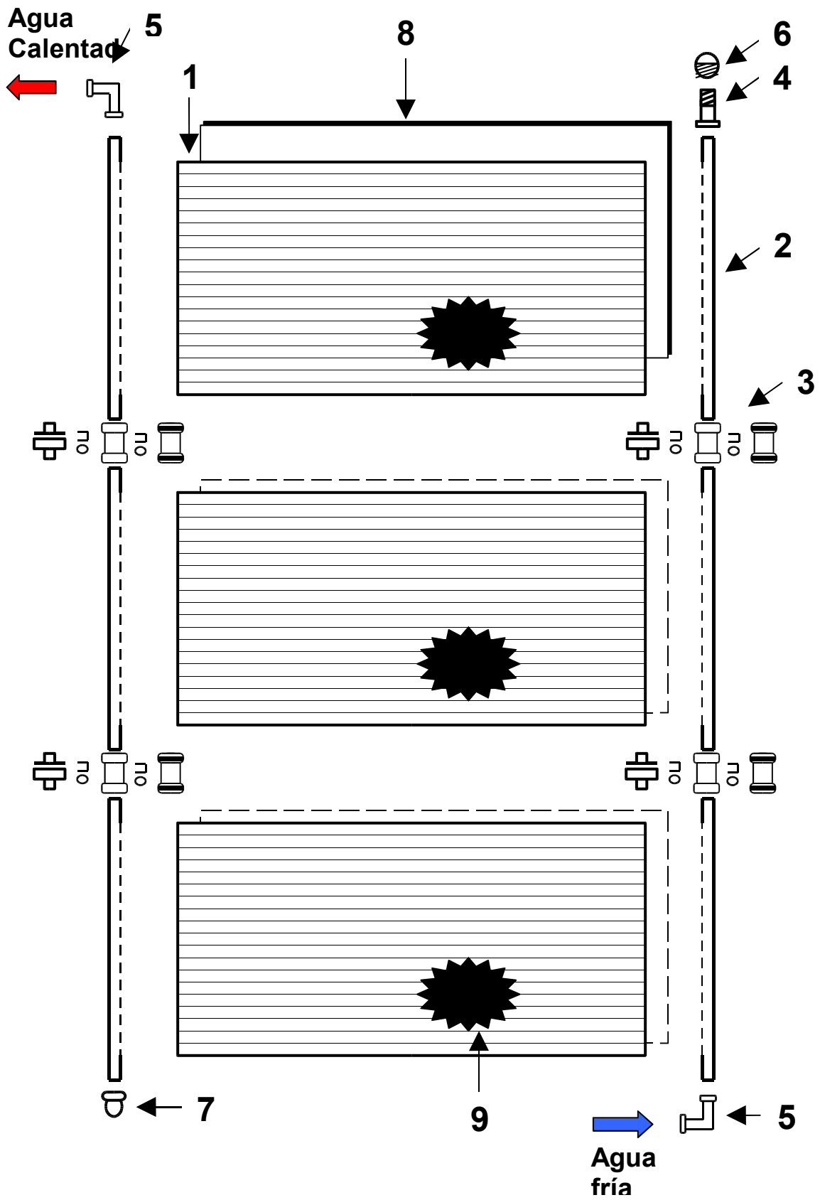
Figura 2. Visualización de las piezas utilizadas en el montaje de tres colectores CSBC
